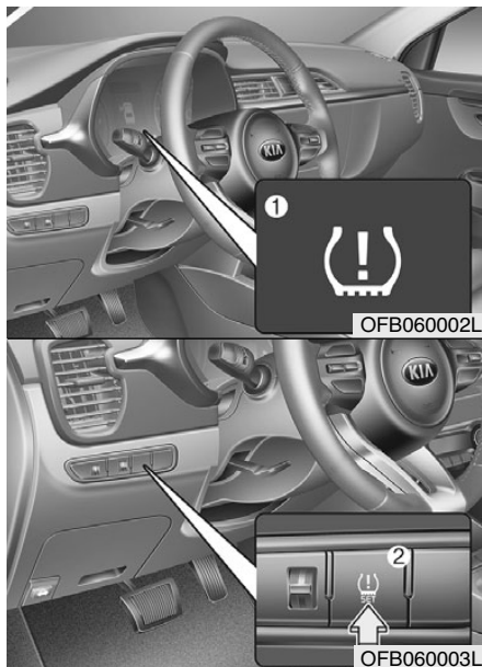
Сигнализатор низкого давления в шине (1)/переключатель настройки системы TPMS (2)
